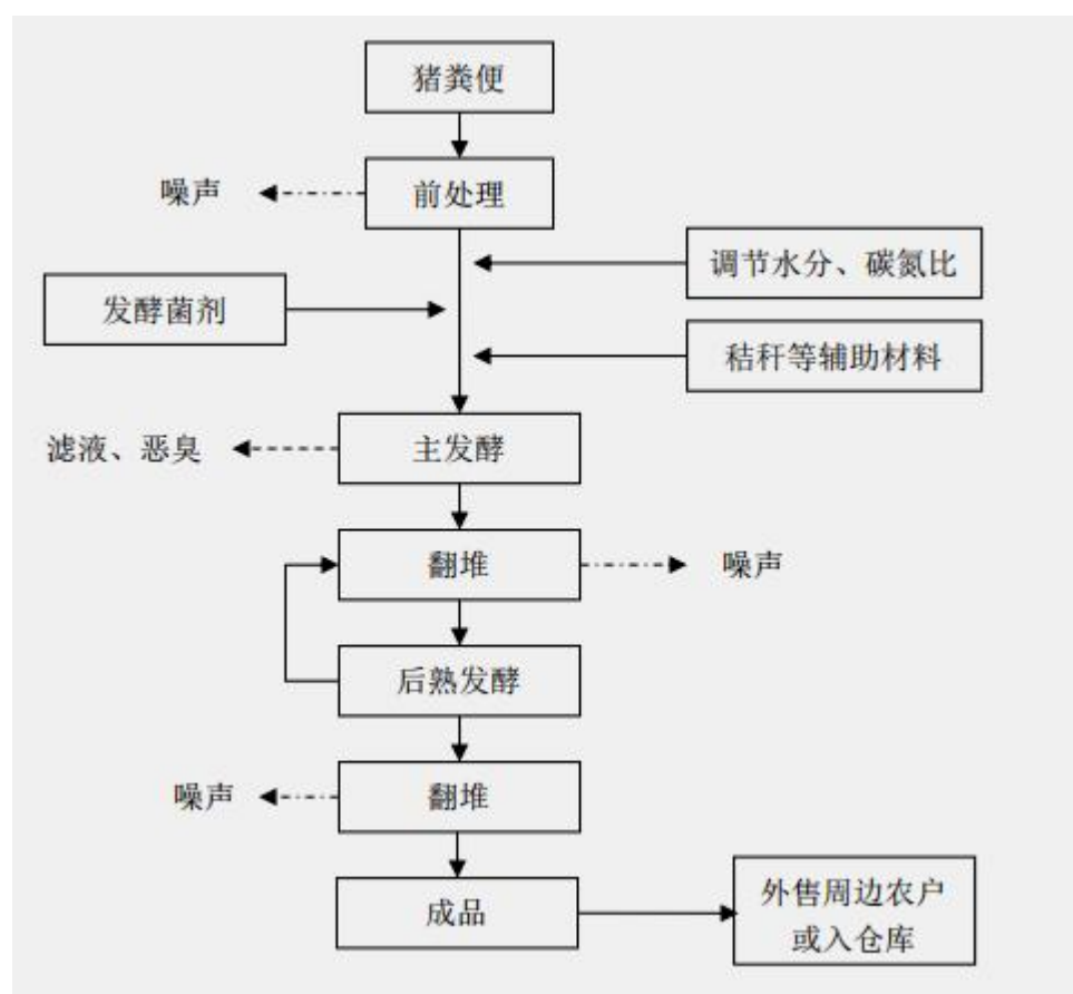
图 3.3.3-1 堆肥工艺流程及产污环节
