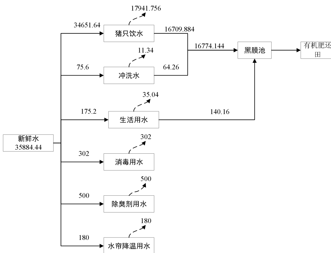
图 3.2.6-1 项目水平衡图 (单位 m³/a)
