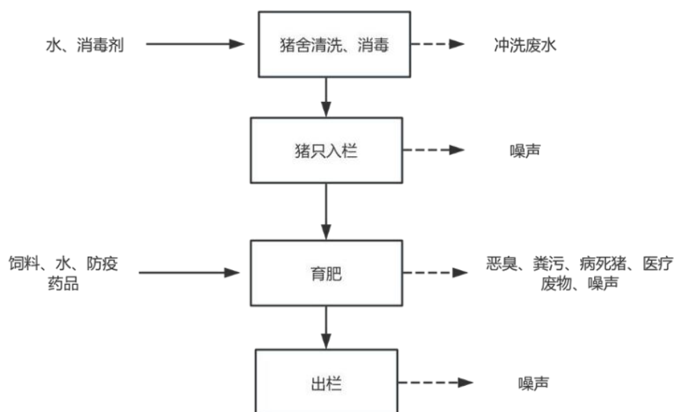
图 3.1.7-1 现有工程工艺流程图
