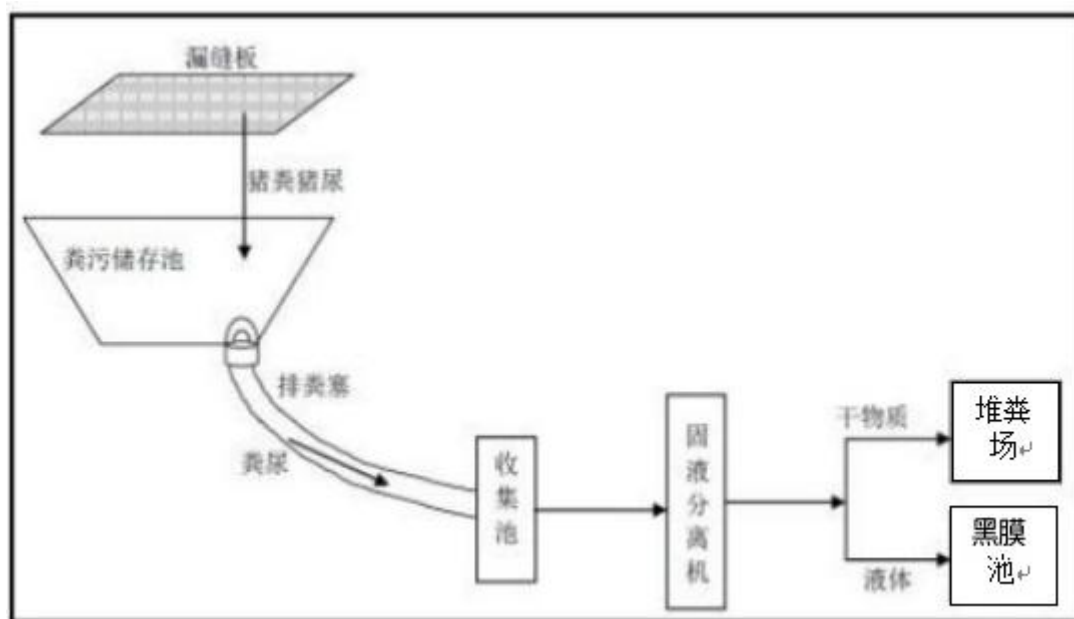
图 3.3.2-1 清粪工艺流程图
