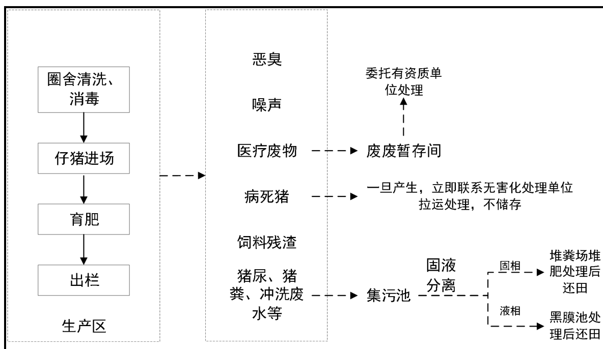
图 3.3.1-1 本项目养殖工艺流程及产污环节图
