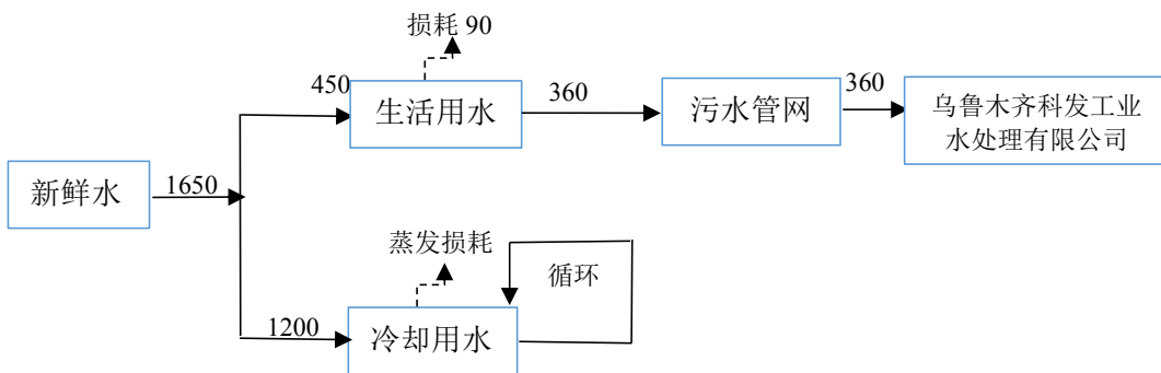
图 2-1 本项目水平衡图 单位：立方米/年
