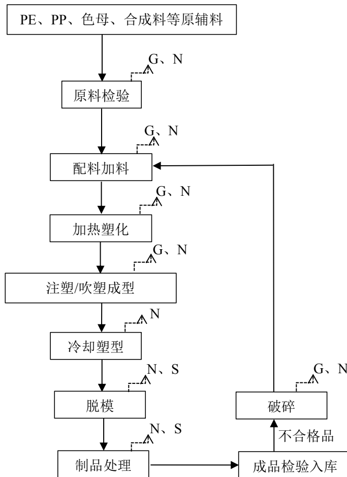
图 2-3 本项目生产工艺流程及产排污环节图
