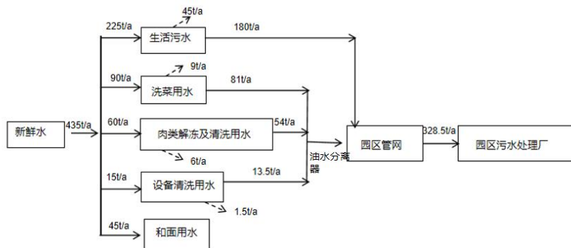
图 2-1 项目水平衡一览图
