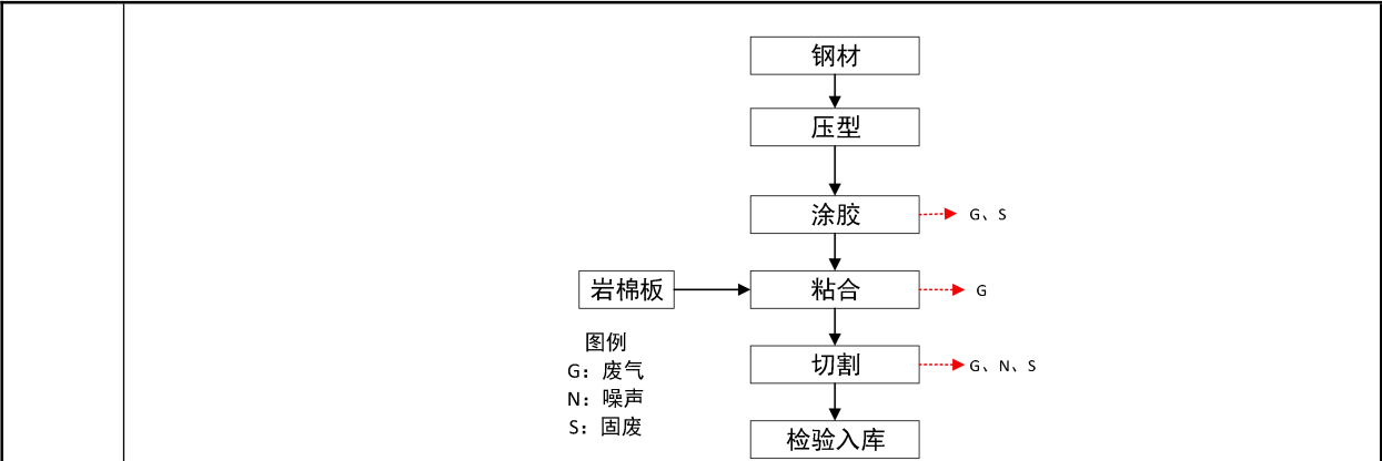
图 2-4 彩钢板生产工艺流程及产污环节图
