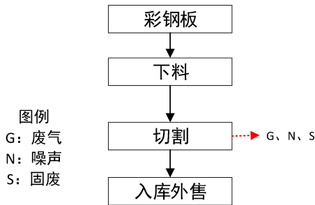
图 2-5 彩钢瓦生产工艺流程及产污环节图
