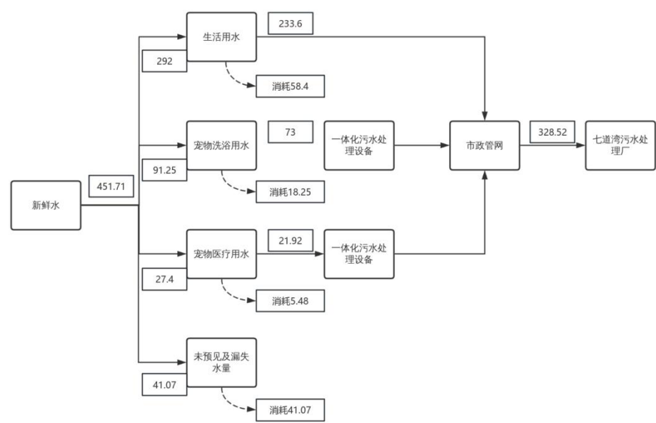
图2-1 本项目水平衡图 单位m 3 /a
