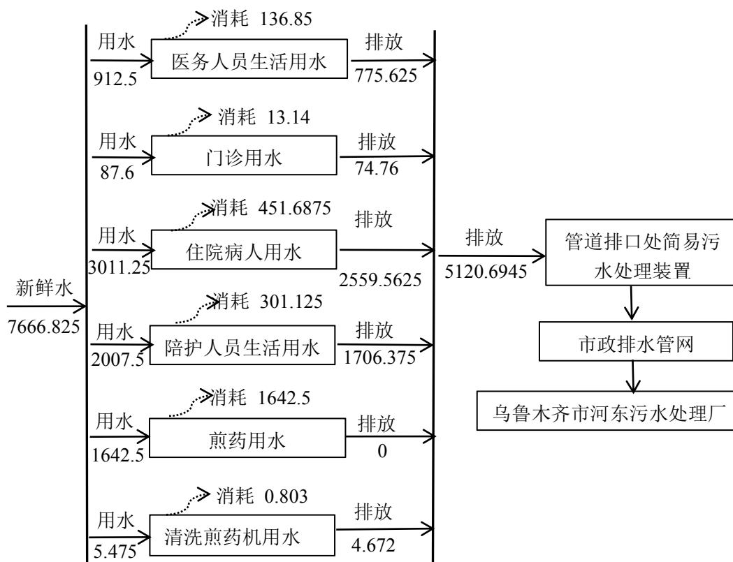
图 2-3 项目水平衡关系图 单位：立方米/年
